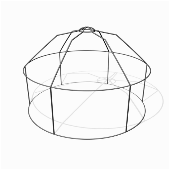
Structure du chapiteau dimensions : Ø :7,50 m – H sous coupole : 4,50 m
